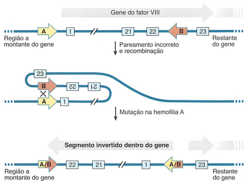
Figura 4-5 Sequências hom logas invertidas, marcadas como A e B, localizadas a 500 kb uma da outra no cromossomo X, uma a montante do gene do fator VIII, e outra em um  ntron entre os  xons 22 e 23 do gene. O pareamento intracromoss mico incorreto e a recombina  o resultam na invers o dos  xons 1 a 22 do gene, interrompendo desse modo o gene e causando hemofilia grave.
